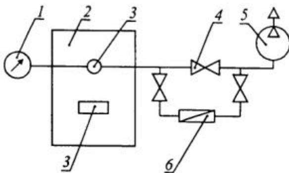
Рисунок 1 — Схема проверки камина на герметичность
