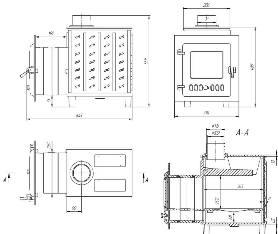
Рис.2 – Общий вид печи
